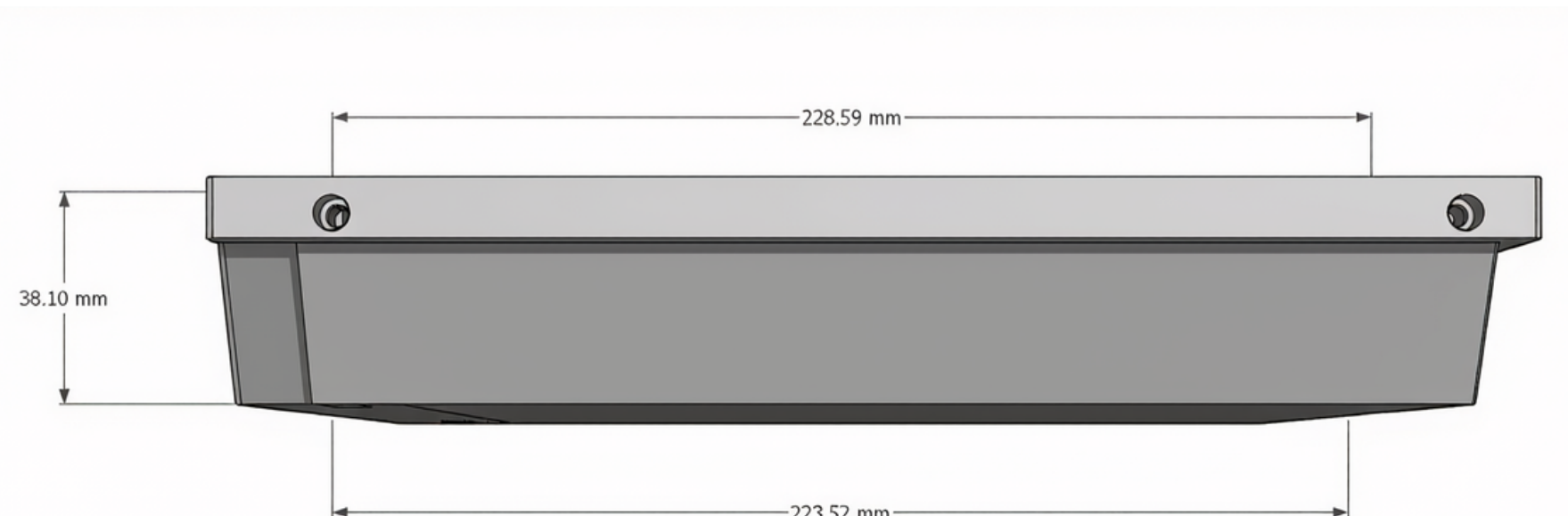
BOTTOM
