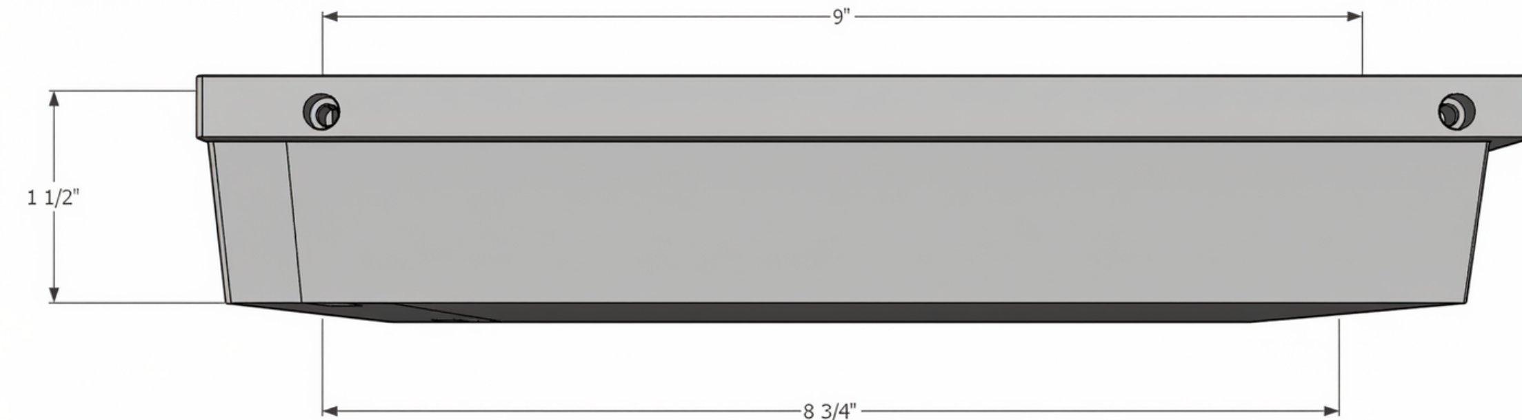
BOTTOM
